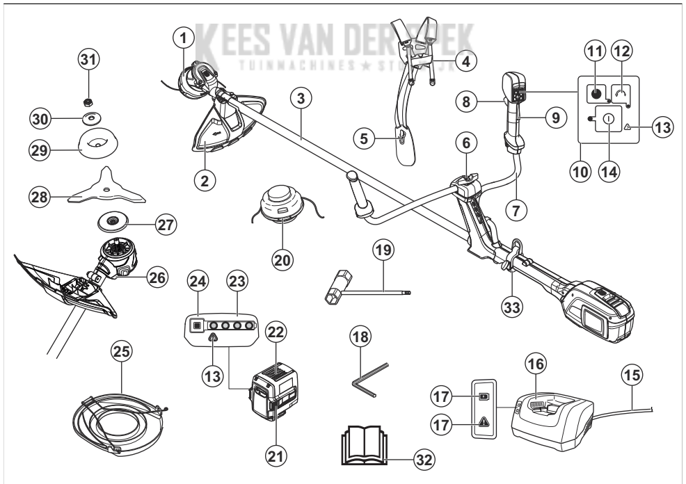
1. Trimmerkopf
