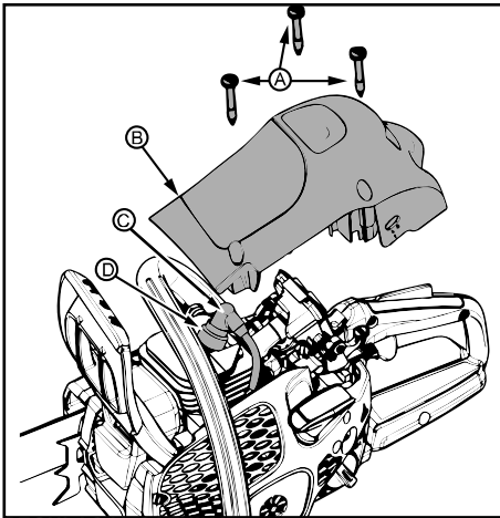
REGULACJA GAŹNIKA
