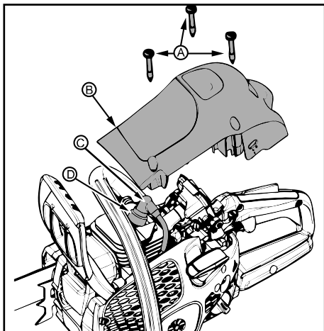
РЕГУЛИРАНЕ НА КАРБУРАТОР
