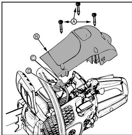
REGLAREA CARBURATORULUI
