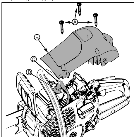
РЕГУЛИРОВКА КАРБЮРАТОРА
