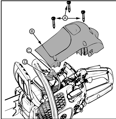
ΡΥΘΜΙΣΗ ΚΑΡΜΠΙΡΑΤΕΡ
